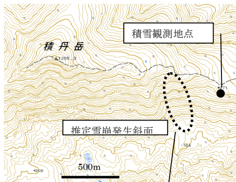
図1 推定雪崩発生斜面付近の地形
