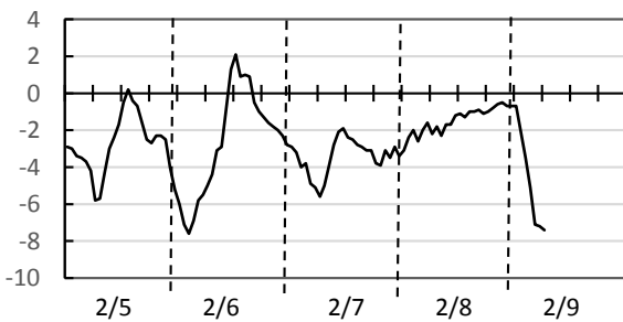
2017/02/05-09石狩アマダス気温
