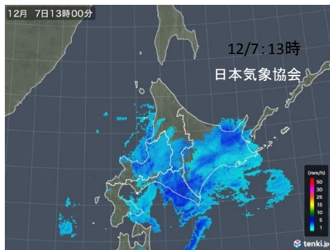
12/7:1時間3mmの降水時
