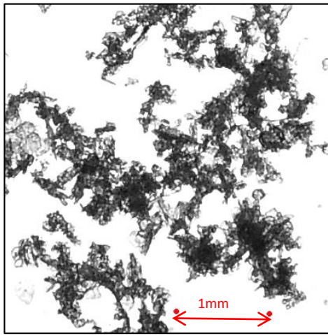
12/7 13:15の降雪 全てが雲粒の集合
