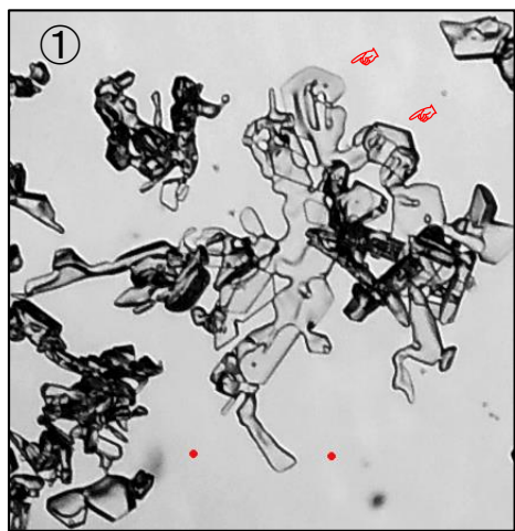
雲粒なし六花 こしもが発達か
