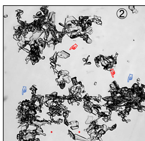
雲粒の塊、「こしも」らしい
