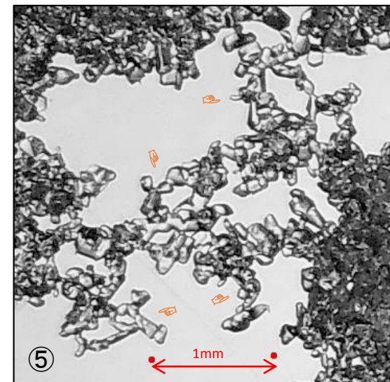
「こしまり」(小さな丸い粒)。一見「新雪」に見える
