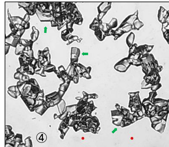
「こしまり」、「こしも」 一見「新雪」に見える
