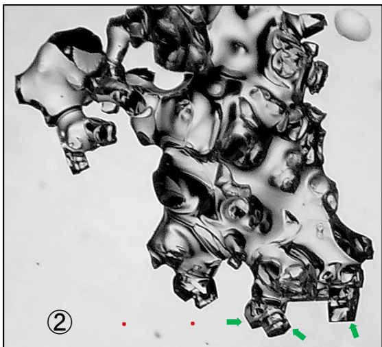
ざらめ (大粒、丸い) 「こしも」形成 →
