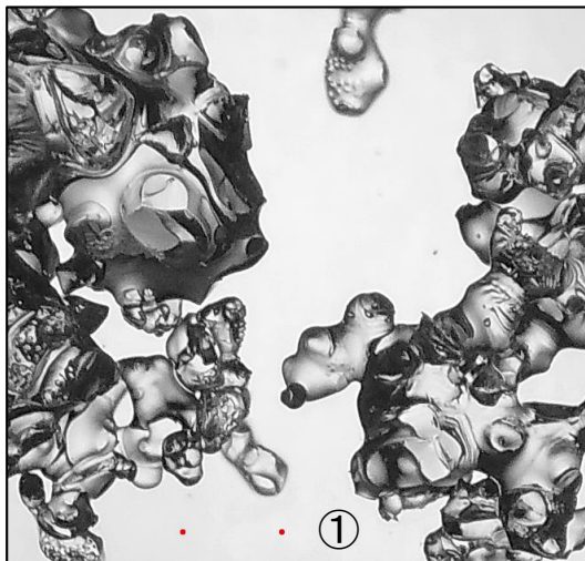
ざらめ (大粒、丸い)
