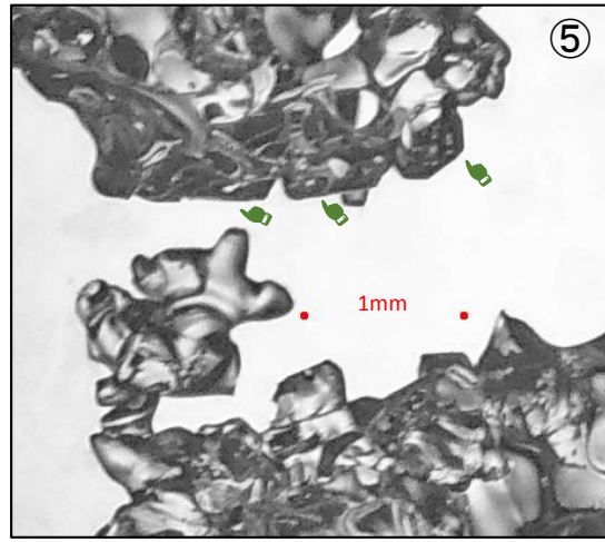
ざらめ・こしも。2/3日の暖気
