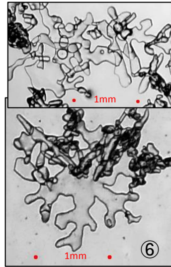
雲粒なし広幅 2/6の降雪
