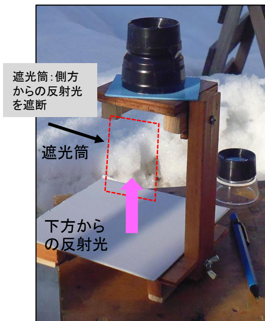
撮影装置外観
